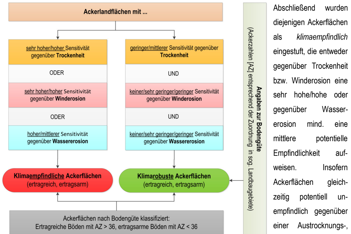
Abbildung 7.15 Herangehensweise zur Identifizierung klimaempfindlicher/klimarobuster Ackerflächen [AZ=Ackerzahl].
